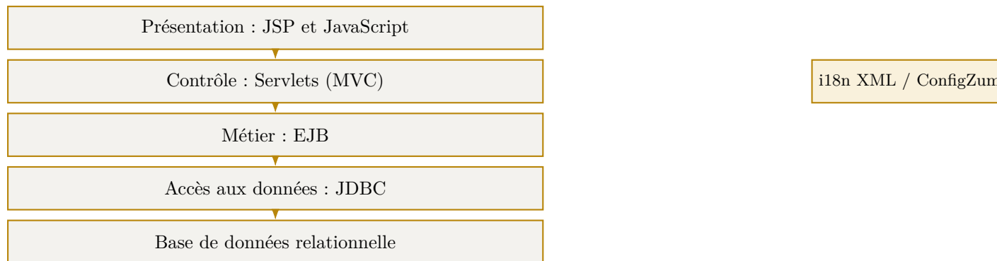
Figure 7.2. Architecture multi-niveaux en couches faiblement couplées.
