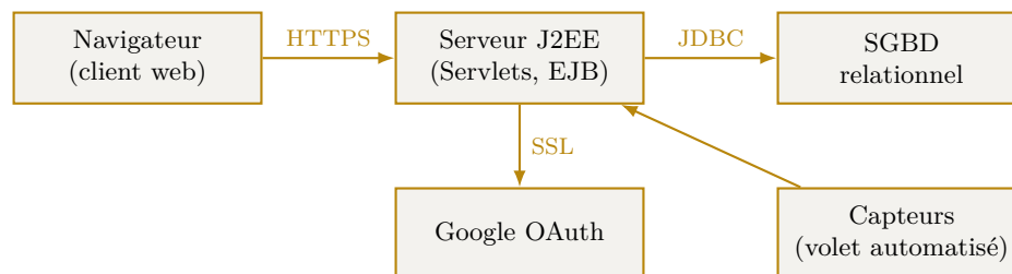
Figure 7.3. Diagramme de déploiement du système.
